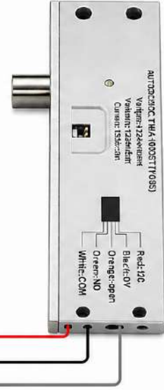
ELEKTROMANYETİK KİLİT
